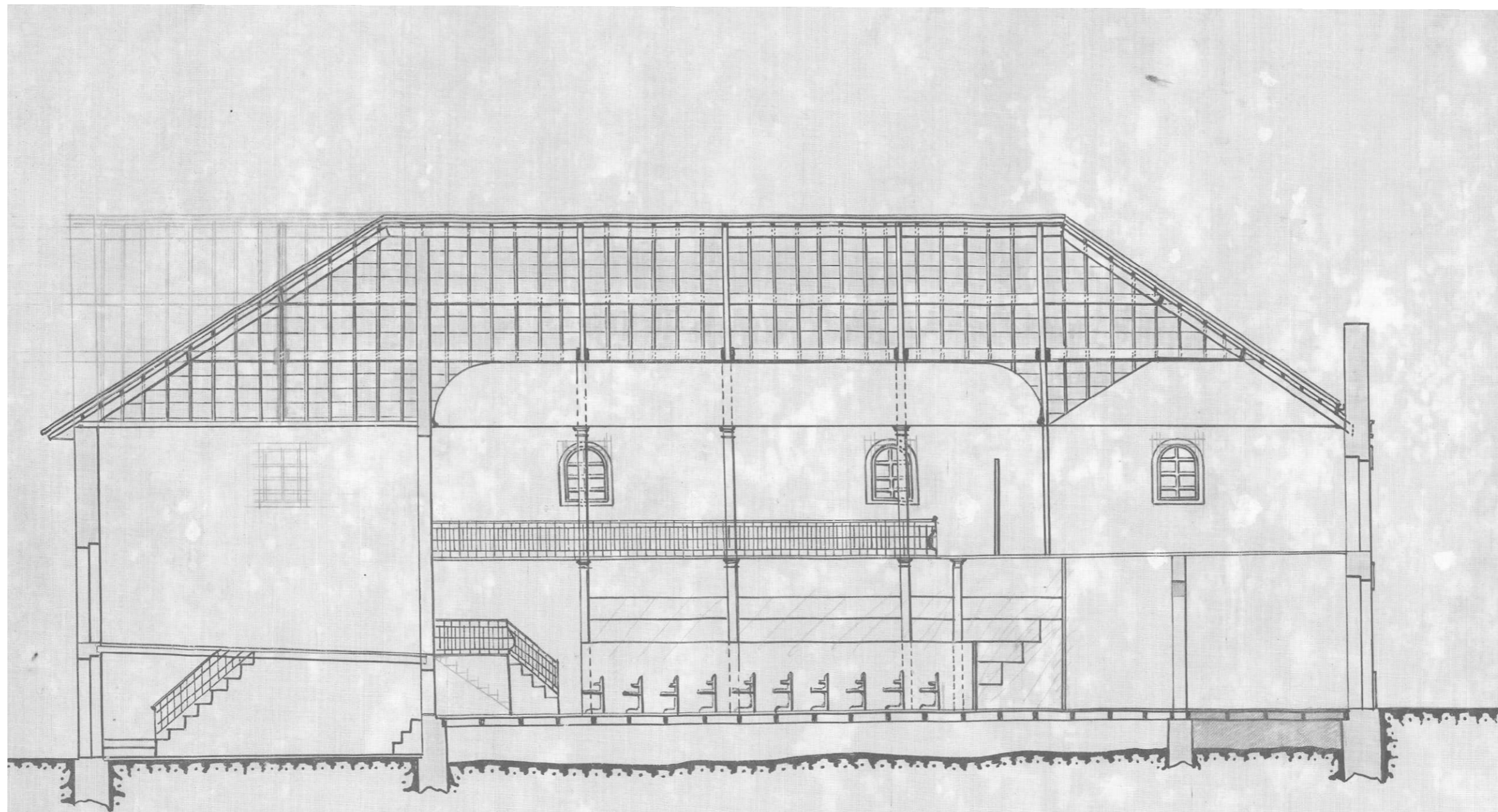
Corte longitudinal pela linha C-D e C'-D'
