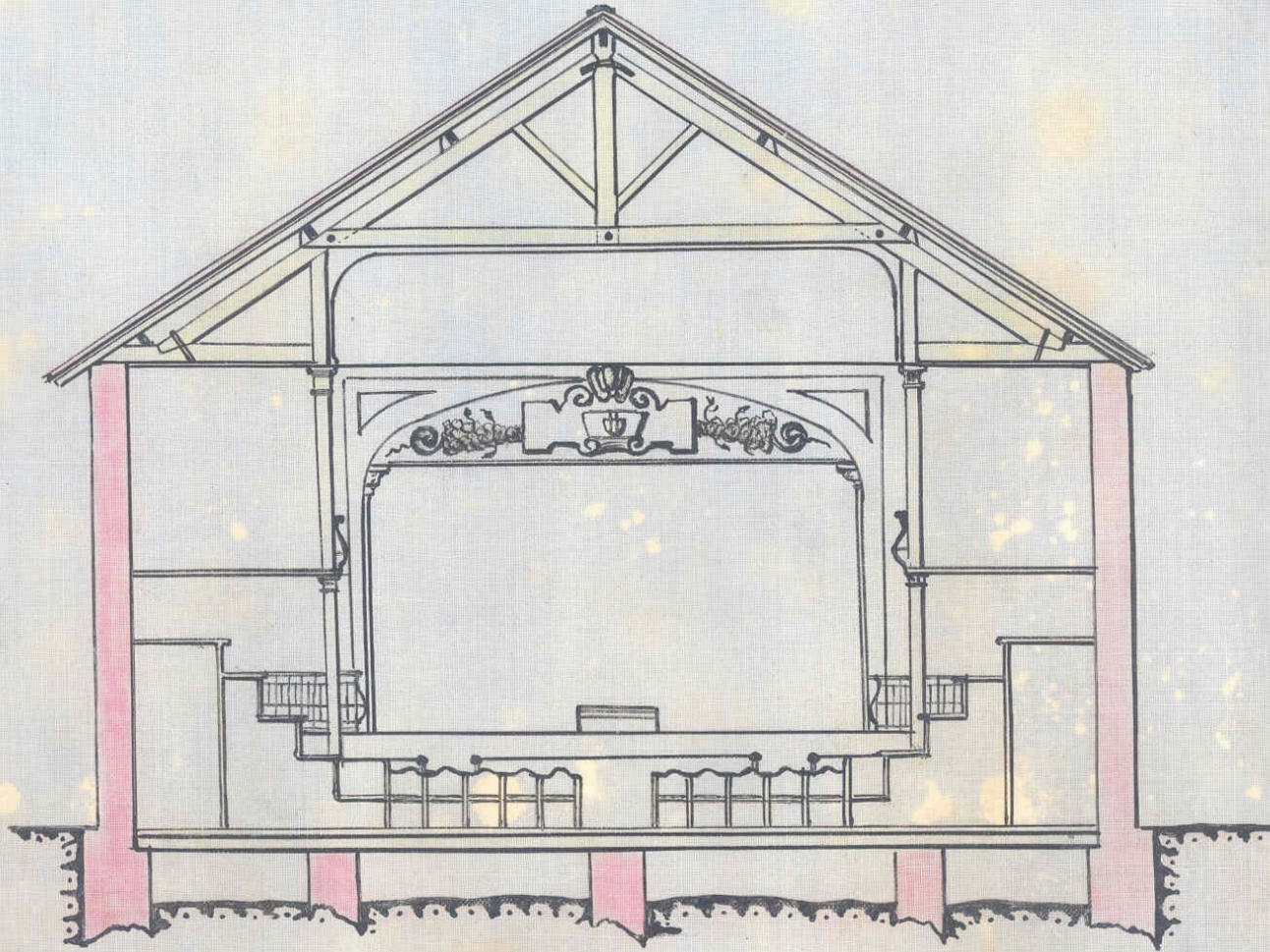
Corte Transversal pela linha A-B-A'B'
